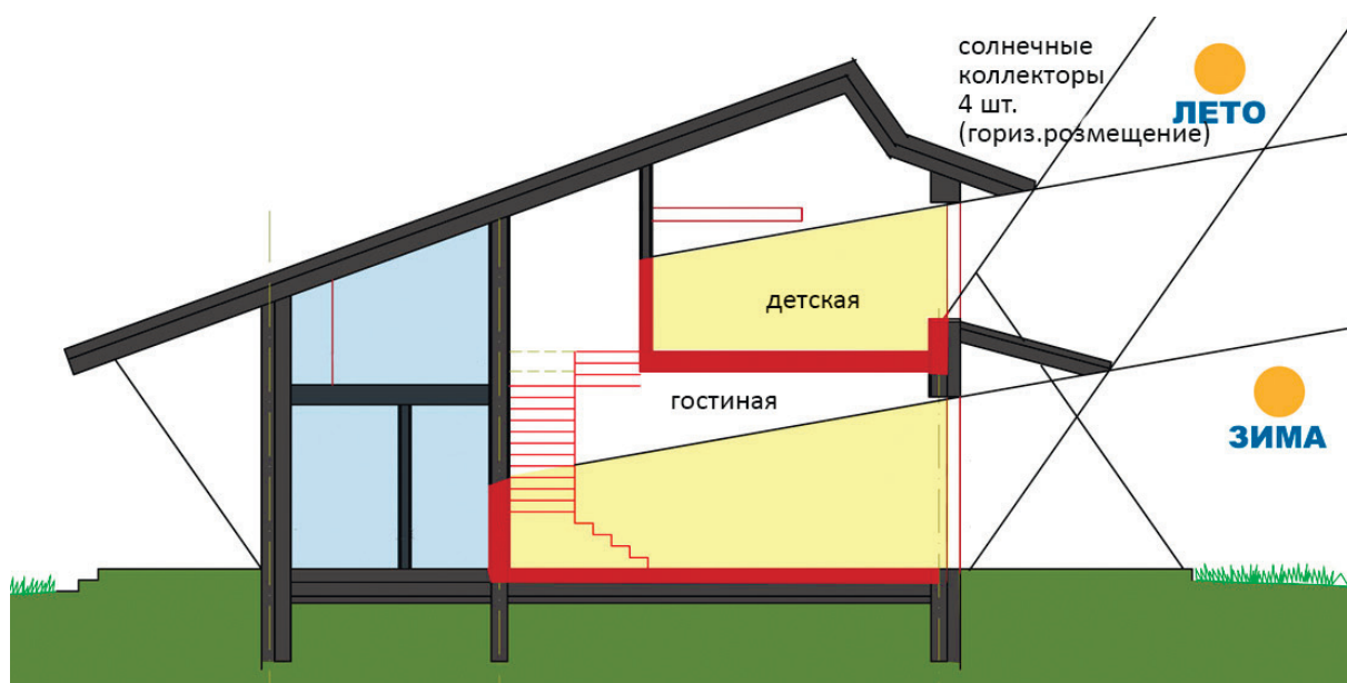
Рис. 3.2.14. Разрез-схема попадания солнечных лучей в дом.
