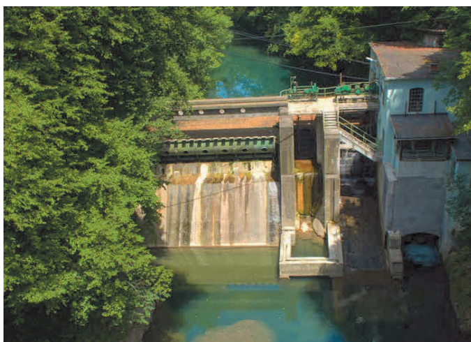
Рис. 3.1.11. Мини-ГЭС на р. Кокра, Словения.
