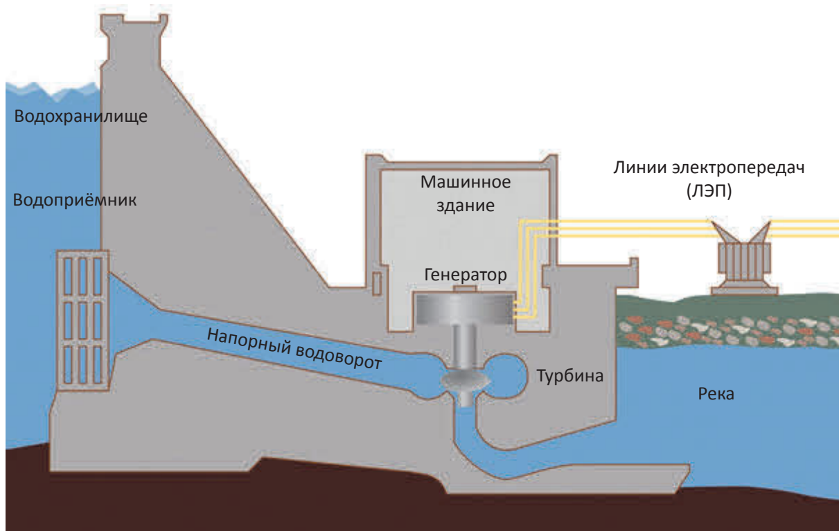
Рис. 3.1.10. Схема плотины гидроэлектростанции (ГЭС).
